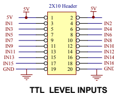
TTL LEVEL INPUTS
