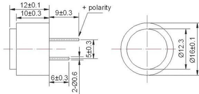
产品尺寸图单位: mm
